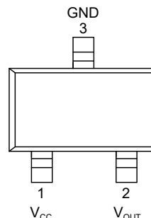
图 4 引脚定义 (SOT23-3)
