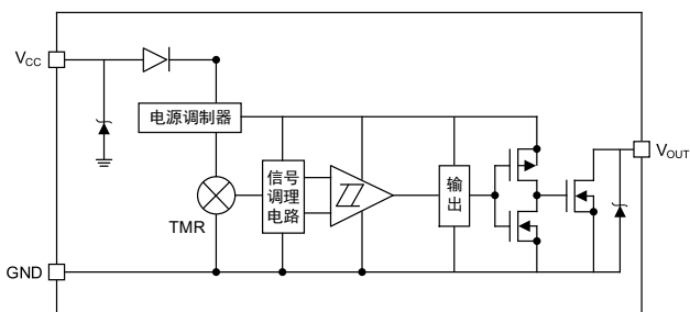
图 1 芯片内部原理框图
