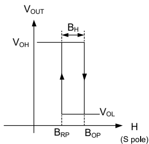
图 3 芯片磁场响应曲线
