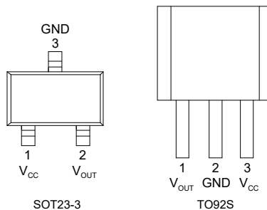
图 4 引脚定义
