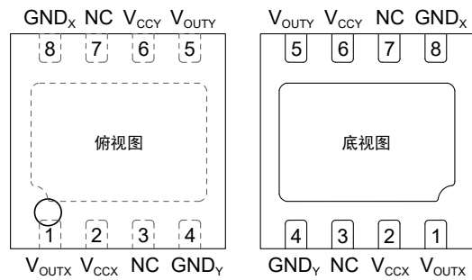
图 4 引脚定义 (DFN8L)
