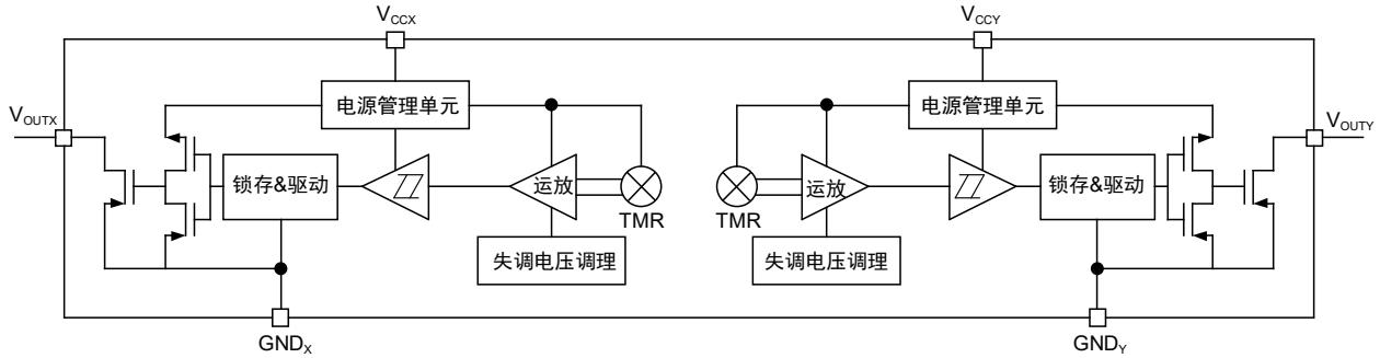
图 1 芯片内部原理框图
