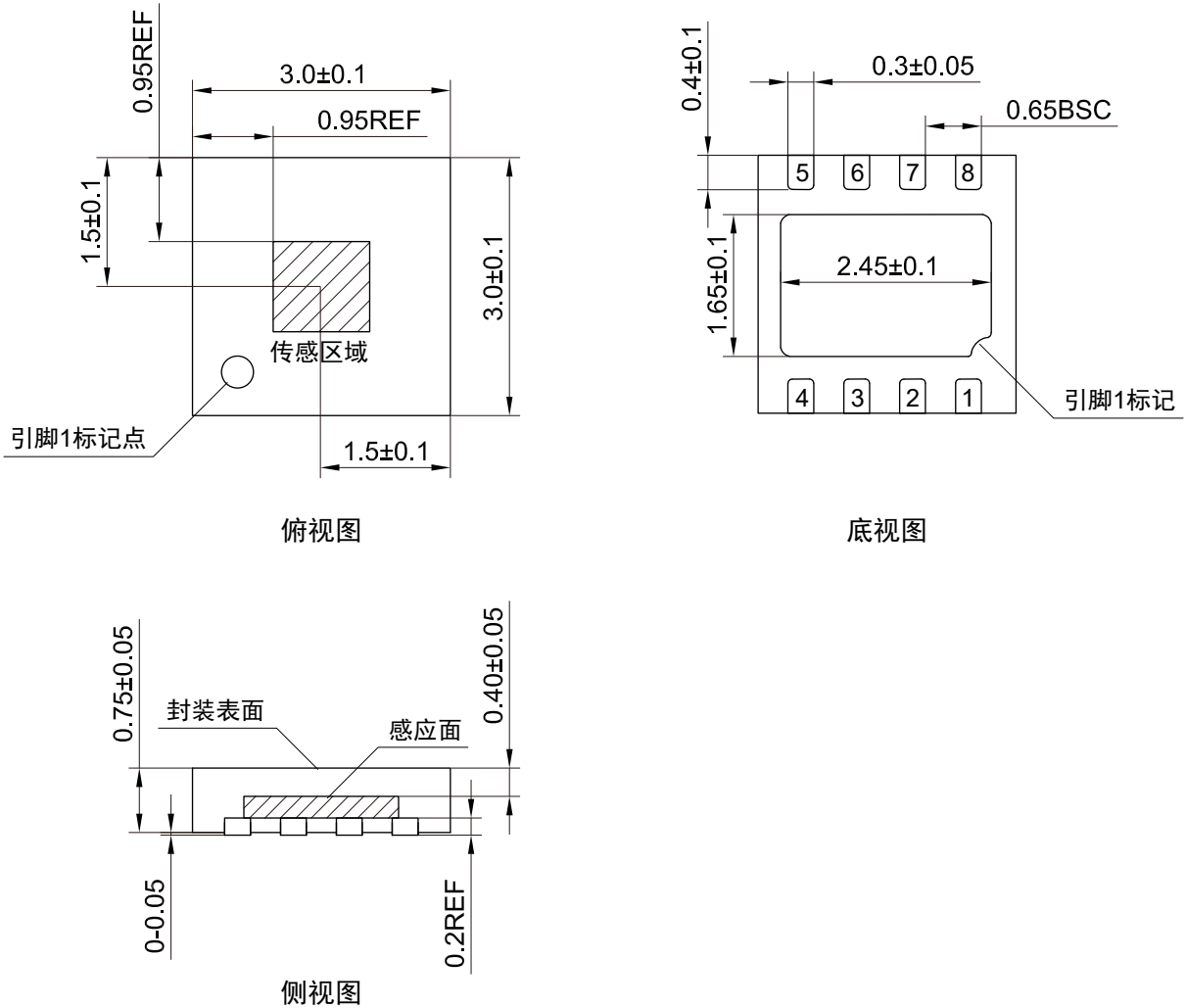
图 10 DFN8L 封装图 (尺寸单位: mm)
