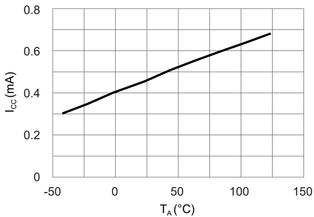
图7 工作电流和工作温度的关系 ( V_{CC} = 12\text{V} )
