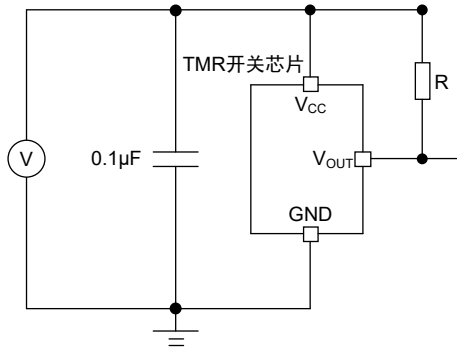
图 9 滤波电容用以降低供电噪音
