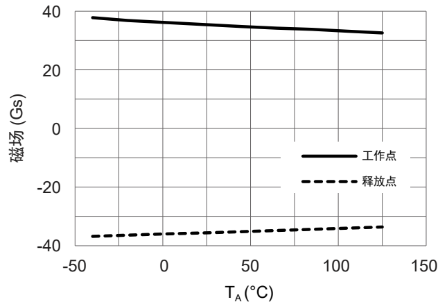
图8 工作点、释放点和工作温度的关系 ( V_{CC} = 12\text{V} )
