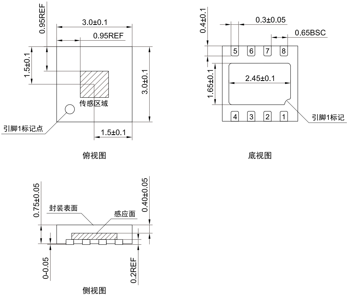
图 15 DFN8L 封装图 (尺寸单位: mm)
