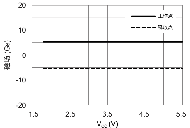
图 8 工作点、释放点和供电电压的关系 ( T_A = 25^\circ\text{C} )
