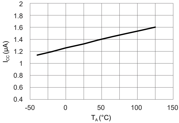
图 9 工作电流和工作温度的关系 (V CC = 3 V)
