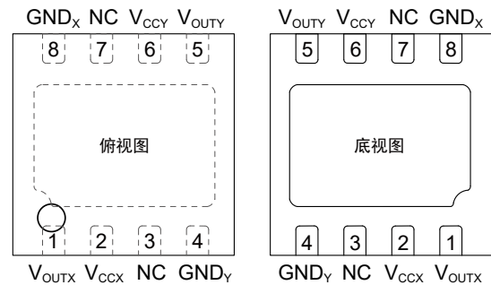
图 4 引脚定义 (DFN8L)
