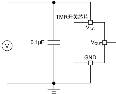
图 13 滤波电容用以降低供电噪音
