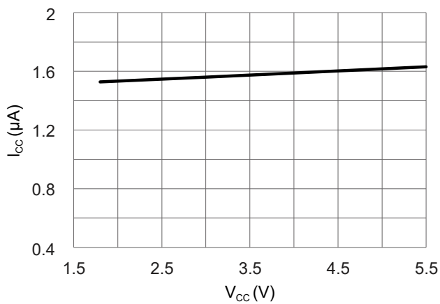
图 7 工作电流和供电电压的关系 ( T_A = 25^\circ\text{C} )
