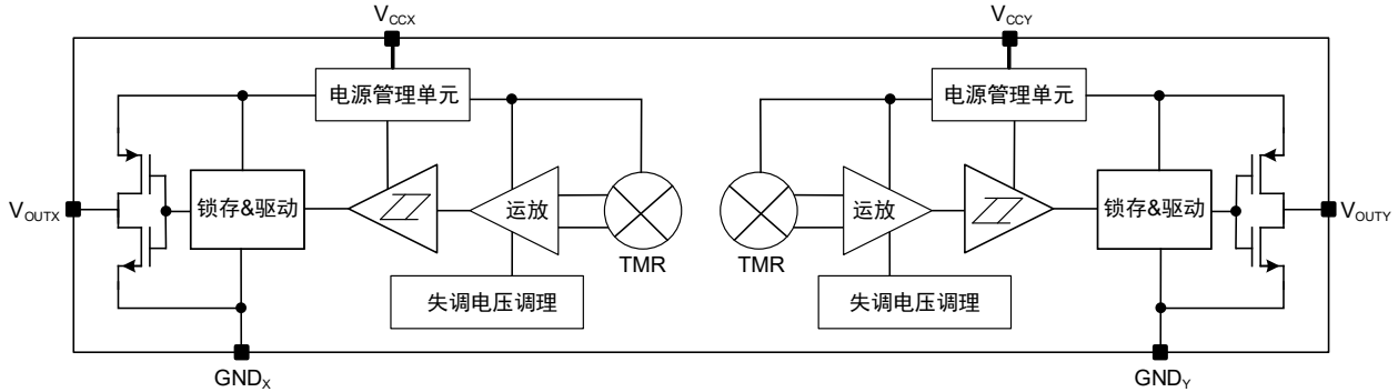
图 1 芯片内部原理框图
