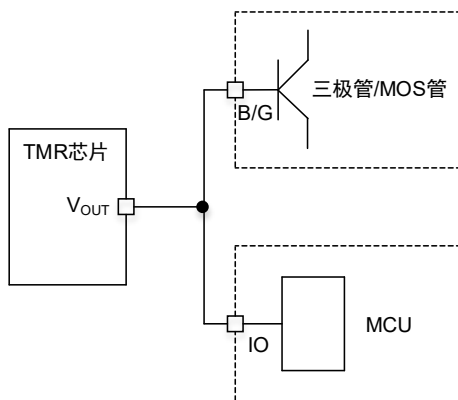
图 14 驱动功率负载的应用电路
