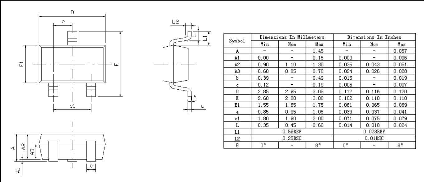
SOT23-3 封装图
