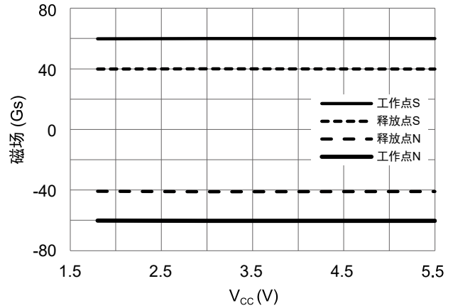
图6 工作点、释放点和供电电压的关系 ( T_A = 25^\circ C )
