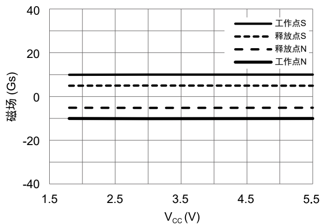
图10 工作点、释放点和供电电压的关系 ( T_A = 25^\circ C )
