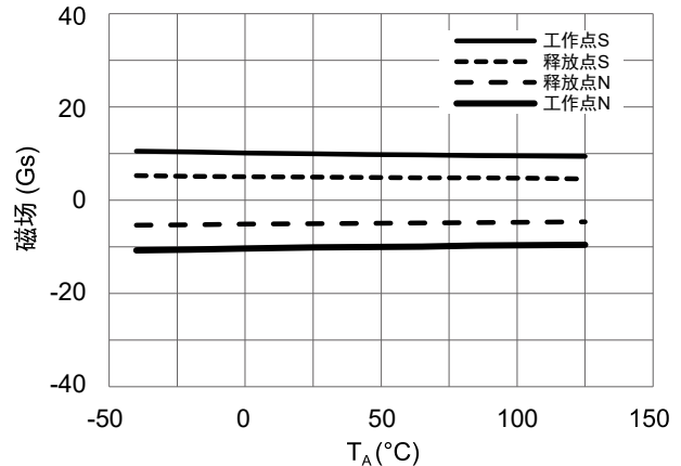
图 16 工作点、释放点和工作温度的关系 (V CC = 3 V)
