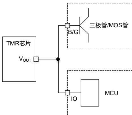
图 18 驱动功率负载的应用电路
