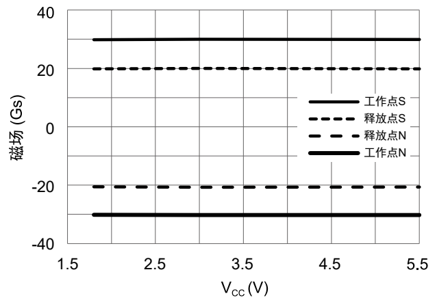
图8 工作点、释放点和供电电压的关系 ( T_A = 25^\circ C )
