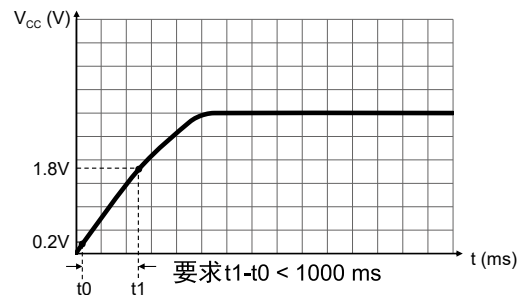
图 19 上电时序图
