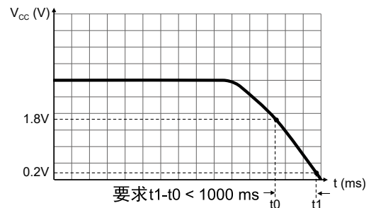
图 20 下电时序图
