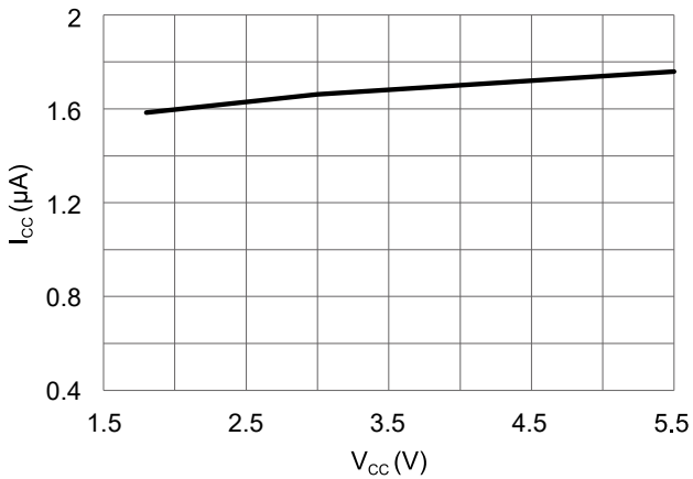
图 11 工作电流和供电电压的关系 ( T_A = 25^\circ C )
