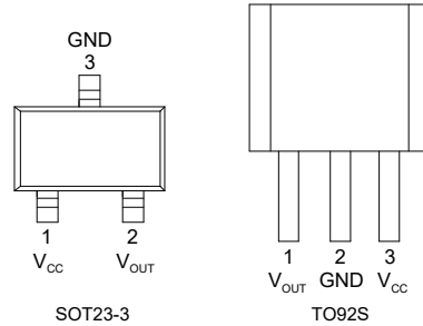
图 4 引脚定义
