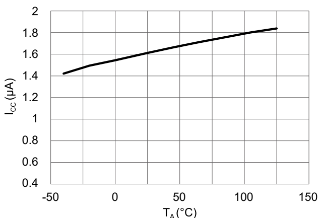
图 21 工作电流和工作温度的关系 ( V_{CC} = 3 V )
