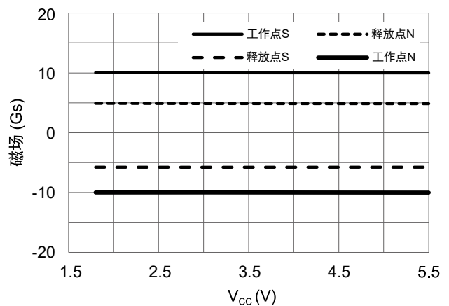
图10 工作点、释放点和供电电压的关系 (T A = 25 °C)
