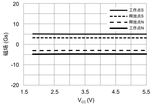
图 12 工作点、释放点和供电电压的关系 ( T_A = 25^\circ C )
