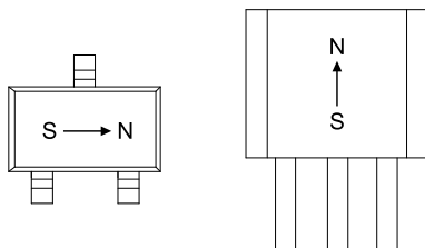
图 2 芯片敏感方向
