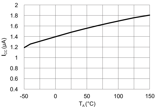
图 15 工作电流和工作温度的关系 ( V_{CC} = 3 V )
