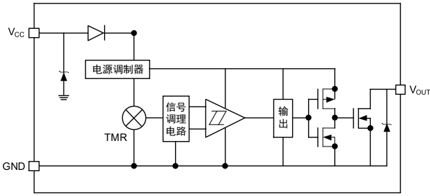
图 1 芯片内部原理框图
