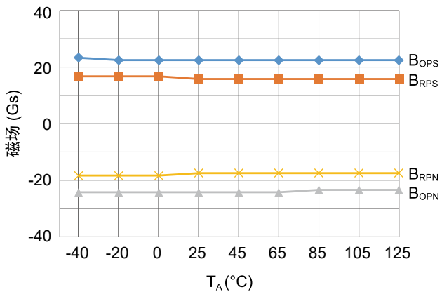
图7 工作电流和工作温度的关系 ( V_{CC} = 24\text{ V} )
