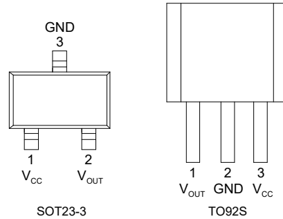
图 4 引脚定义
