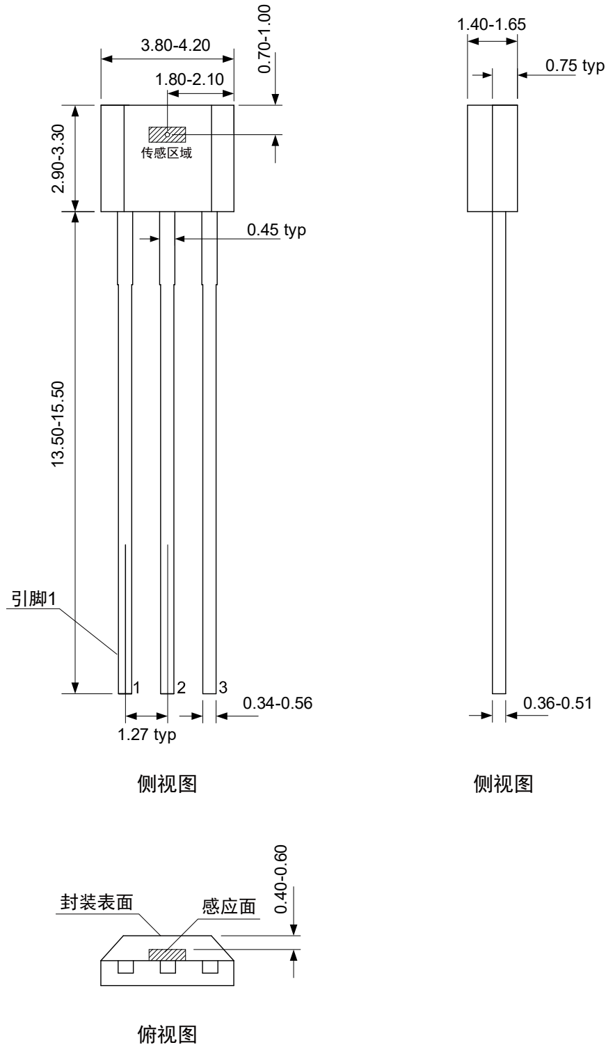
图 11 TO92S 封装图 (尺寸单位: mm)
