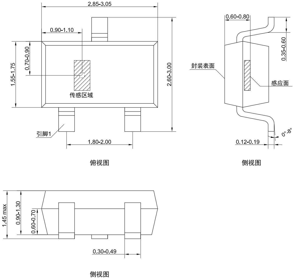
图 10 SOT23-3 封装图 (尺寸单位: mm)
